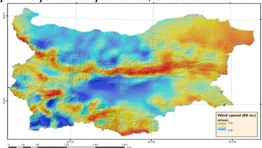
Фигура 14. Теоретичен ветрови потенциал на височина 80 м
